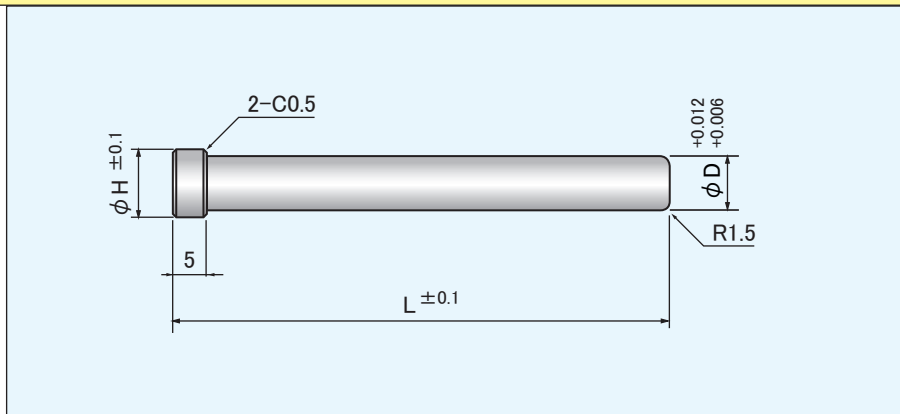
ダウエルピン (DOWEL PINS)
